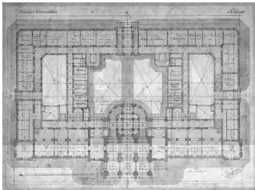
Az új városháza földszinti alaprajza HU-MNL-BKML-XV.15.a. [Tervrajzok gyűjteménye. Kecskeméti épületek tervrajzai, 1835–1999] 185.
